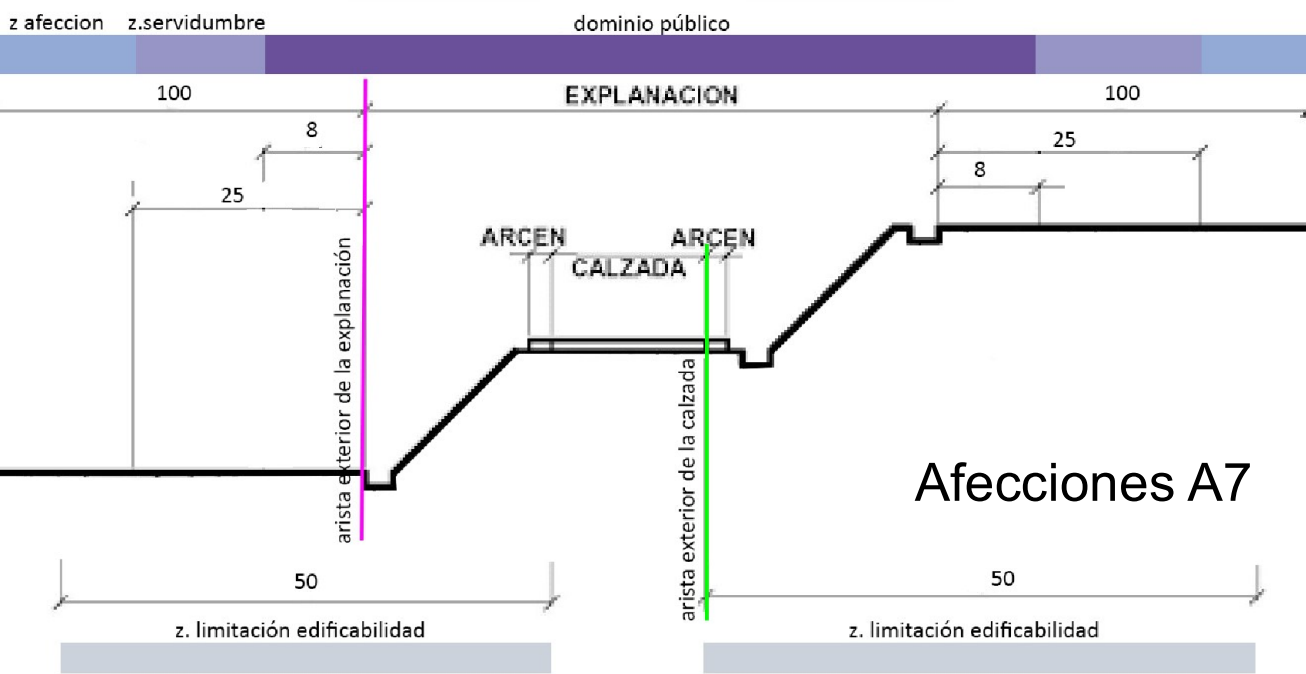
Esquema Afecciones Carreteras
