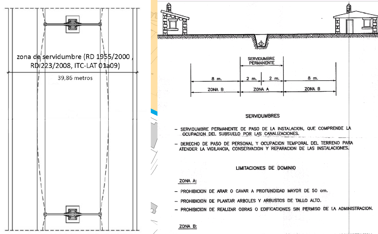
Esquema Afecciones Hidrocarburos e Infrast. eléctricas
